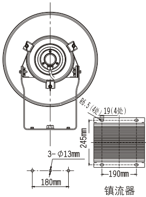
座式安装
